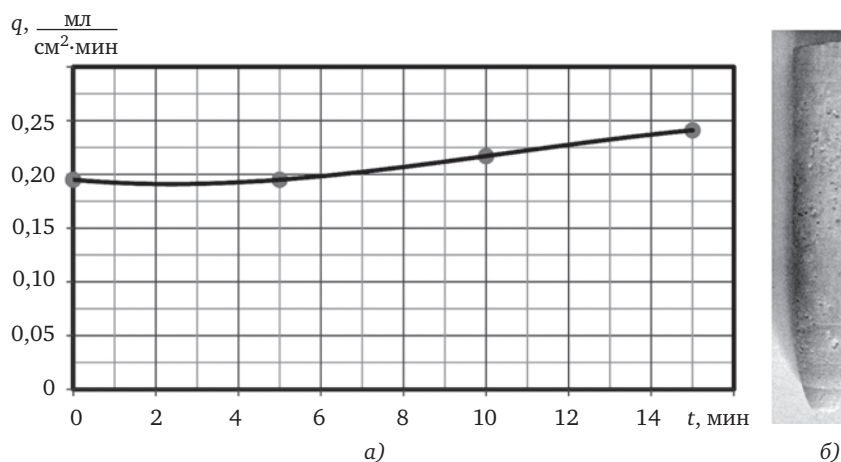
Рис. 5.3. Зависимость удельной газопроизводительности для катода №1 из сплава алюминия с индием и галлием от времени испытания (а) и внешний вид поверхности катода (б)
