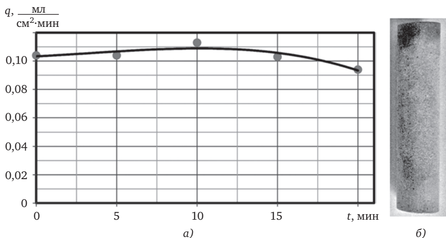
Рис. 5.6. Зависимость удельной газопроизводительности для катода из сплава Д16Т от времени испытания (а) и внешний вид поверхности катода (б). Электролит — водопроводная вода
