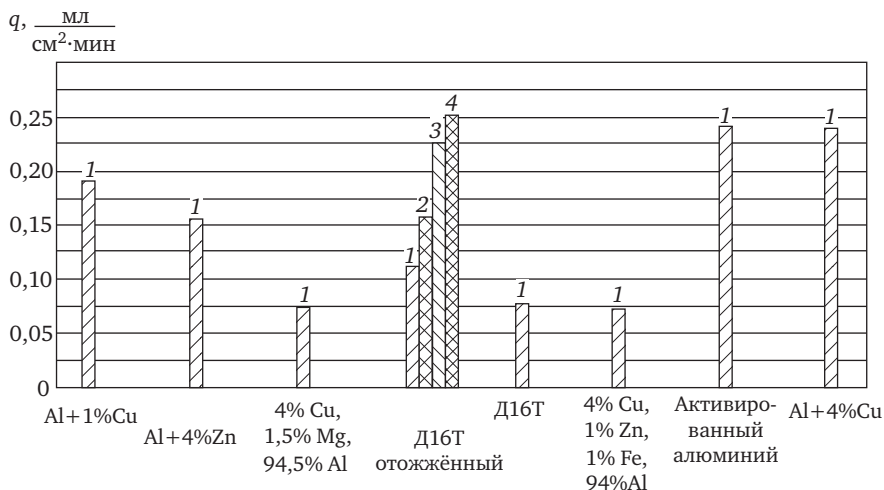
Рис. 5.10. Показатели удельной газопроизводительности для различных катодов.
