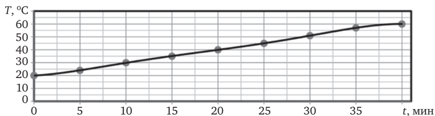
Рис. 5.13. Изменение температуры в электролизной ячейке по времени для катода №3 (4% Cu, 1% Zn, 1% Fe, 94% Al). Электролит — водопроводная вода
