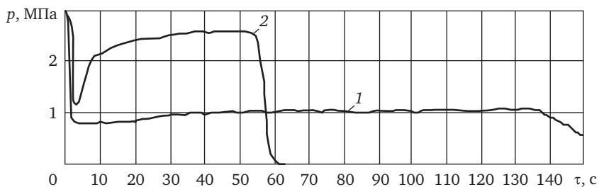
Рис. 3.2. Пример регулирования газогенератора водорода на металлизированном топливе ТГТ-5:
