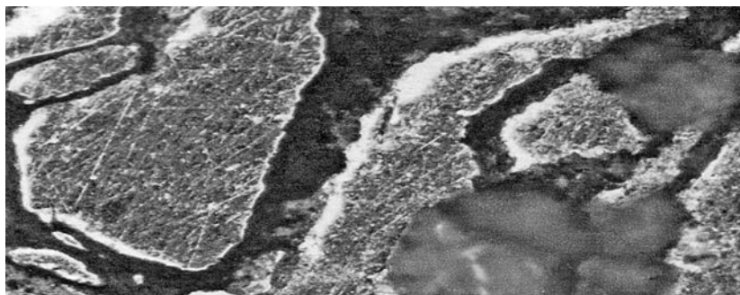
Рис. 9.8. Шлиф прессованного образца стружки сплава АМг-6 с NaOH; светлые фрагменты — АМг-6, темные включения — NaOH. Увеличение 100х
