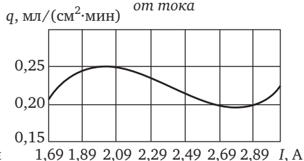
Удельная газопроизводительность от тока
