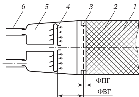
Рис. 2.3. Схема газогенератора:
