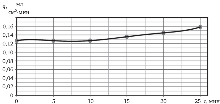
Рис. 5.7. Зависимость удельной газопроизводительности для катода из сплава Д16Т от времени испытания. Электролит — вода с содержанием морской соли 3,5 г/л
