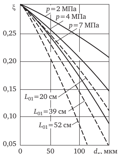
Рис. 2.9. Относительная доля осевших частиц металла в зависимости от их диаметра d_k , длины зоны горения L_{01} и давления p
