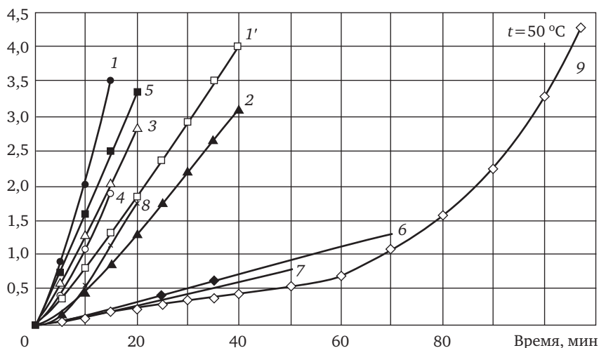
Рис. 9.2. Газопроизводительность по водороду для различных алюминиевых сплавов в растворе 0,1 Н NaOH:
