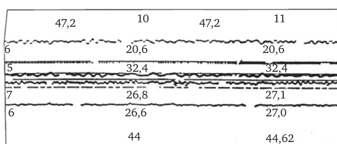
Рис. 2.1. Пример нормального горения ЭАВ (ГРТТ) с водой (копия осциллограммы)
