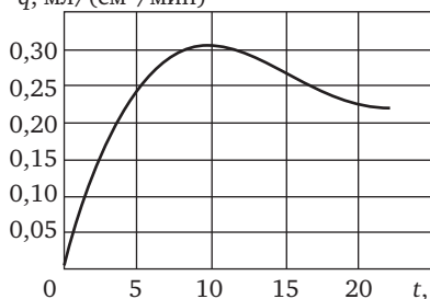
Удельная газопроизводительность
