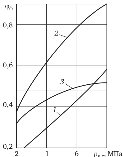
Рис. 2.11. Фактическая полнота сгорания \varphi_\phi алюминия (1) и углерода (2) без потерь и алюминия с осаждением на стенку камеры сгорания (3)
